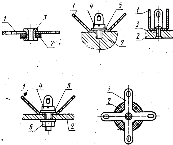
1—лепесток; 2—основание; 3—заклепка; 4—винт; 5—шайба; 6—гайка.
